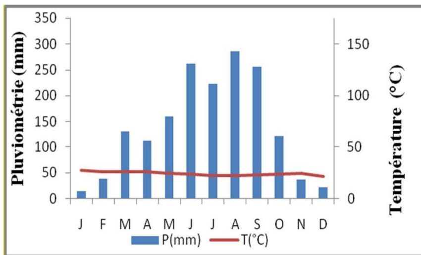
Figure 10 : Diagramme ombrothermique de la station d'Atakpamé (Région des Plateaux) (Moyenne de 2000 à 2018)
