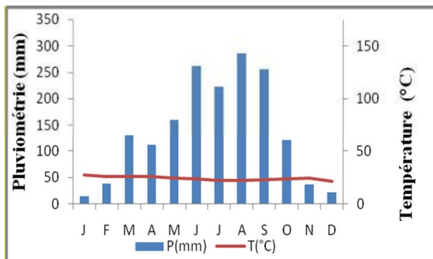
Figure 7 : Diagramme ombrothermique de la station d'Atakpamé (Région des Plateaux) (Moyenne de 2000 à 2018)
