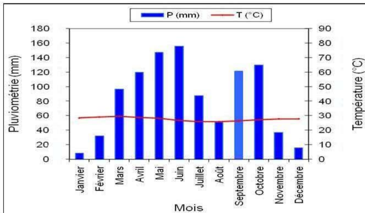
Diagramme ombrothermique de GAPE-CENTRE
