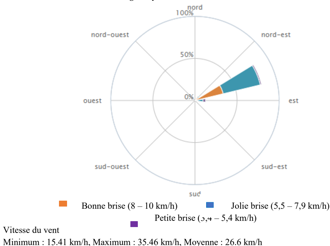
Figure 3: Rose des vents de la Région maritime
